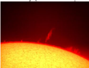
Protuberanzen am 3.10.2007
